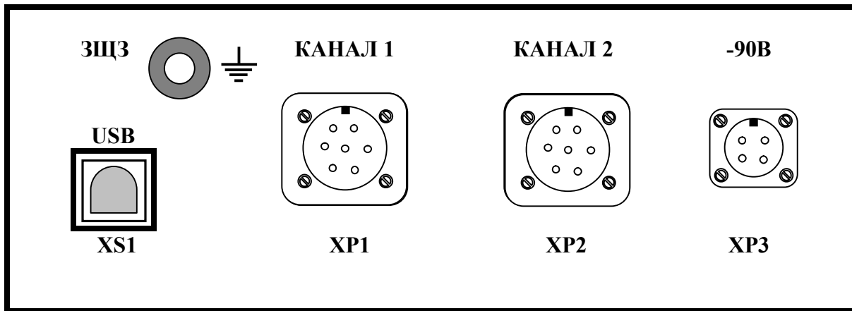
Рис. 2 Задняя панель МТС-2ТМ-USB/М-Т.
